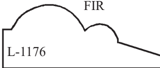
BEVEL BASE CAP 5/8 x 1-5/8 FIR
